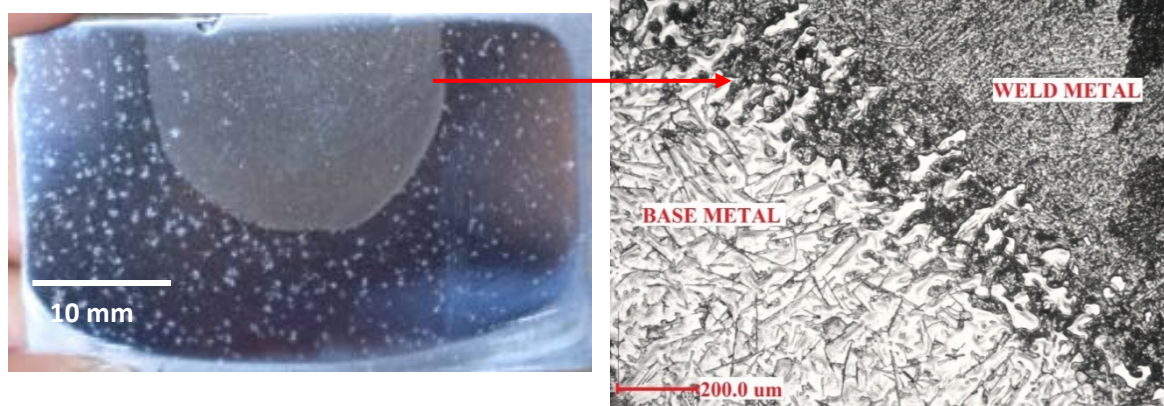
Gambar 5. Permukaan spesimen hasil perbaikan dengan menggunakan metode CFC Closed Mold dan struktur mikro (Hasil poin 10 di Tabel 1)
